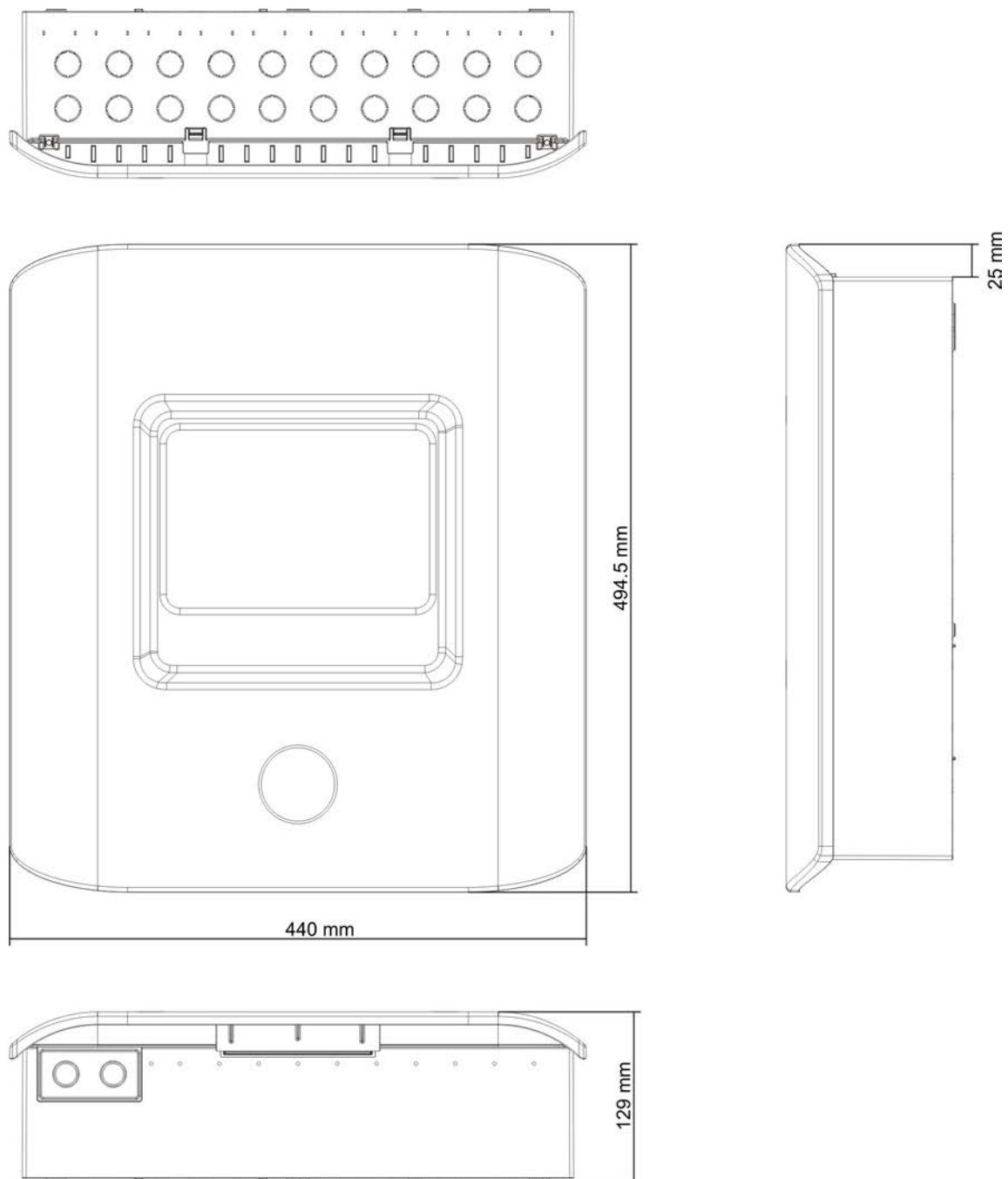
Figura 23: Módulo de ocho zonas con cubierta
