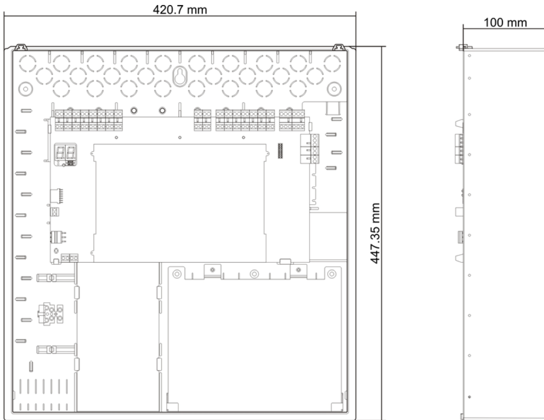
Figura 24: Módulo de ocho zonas sin cubierta
