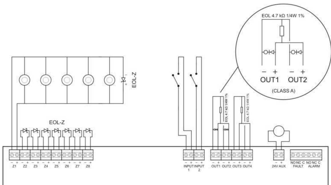
Figura 5: Conexiones del sistema de detección EN 54-13
