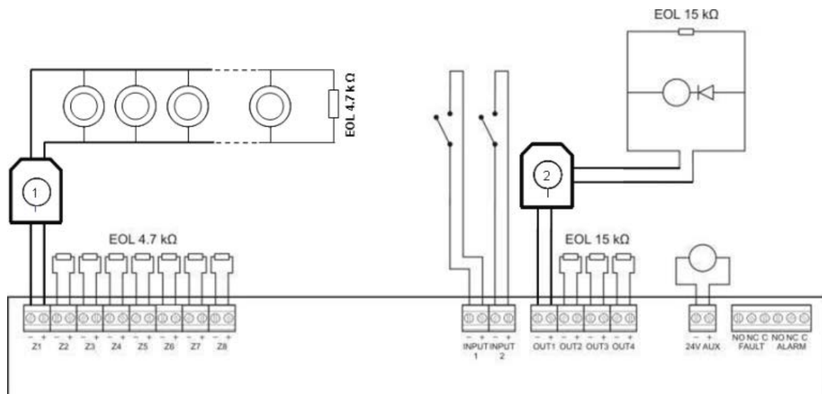
Figura 7: Conexiones del sistema de detección intrínsecamente seguro
