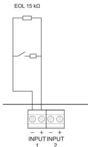
Figura 8: Conexión de las entradas supervisadas
