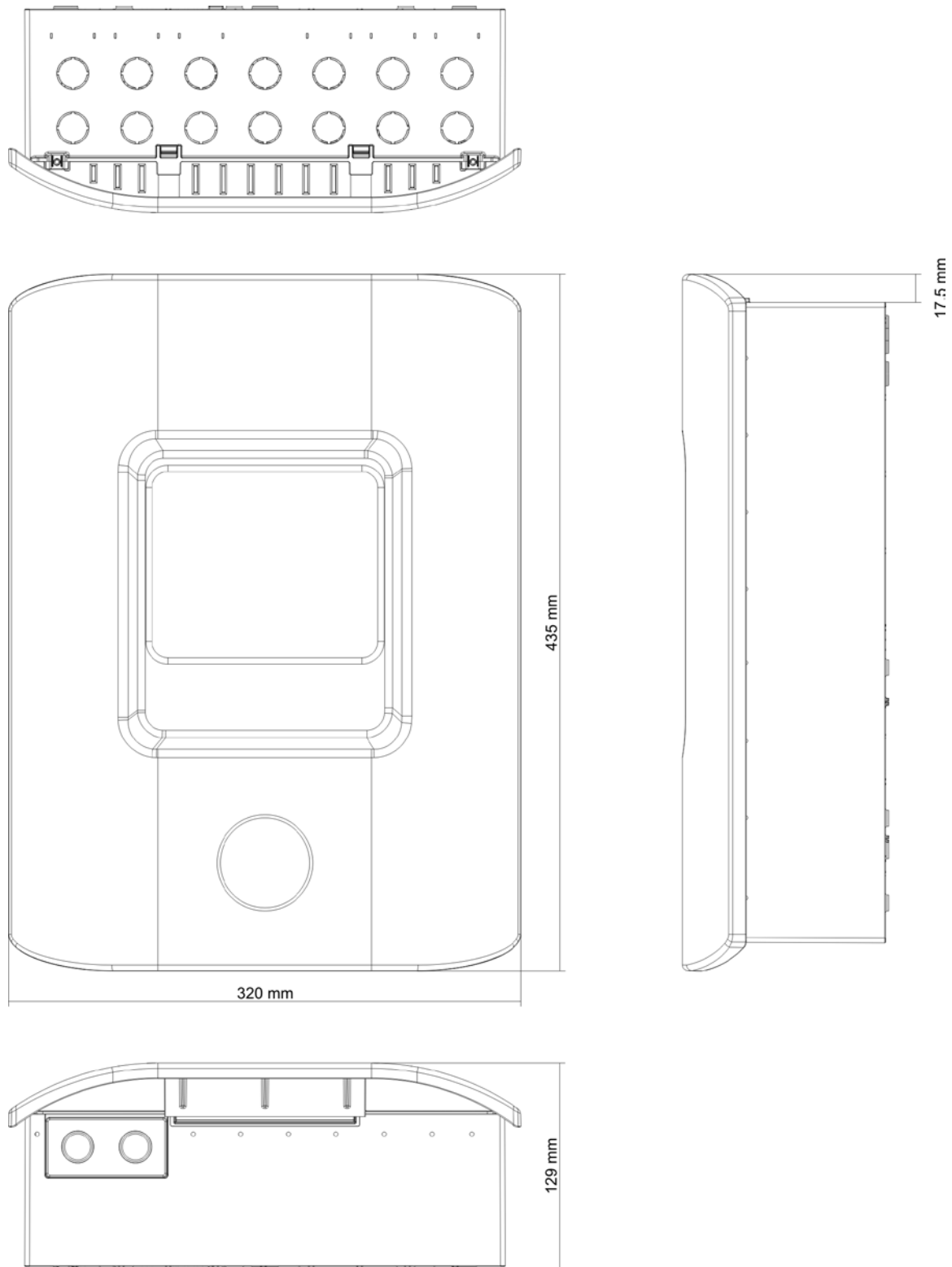
Figura 21: Módulo de dos y cuatro zonas con cubierta
