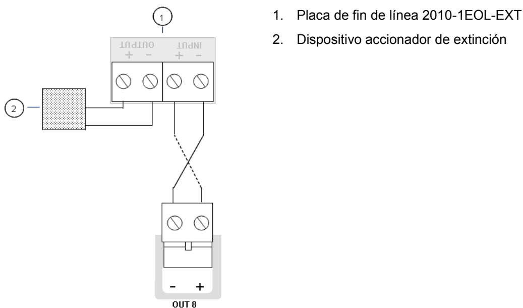
Figura 7: Conexión del accionador de extinción en la central
