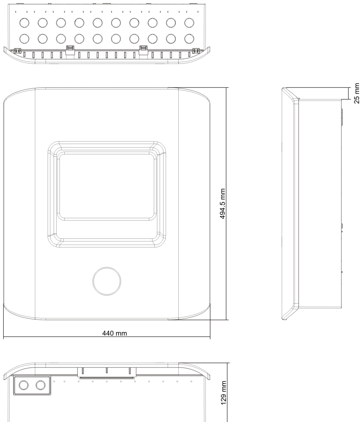
Figura 18: Módulo de la central con cubierta
