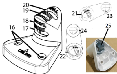
Figura 3: Instalación del soporte de montaje SB100
