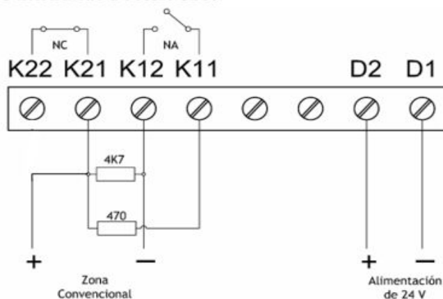
CABLEADO BARRERA C-9105R GST:
